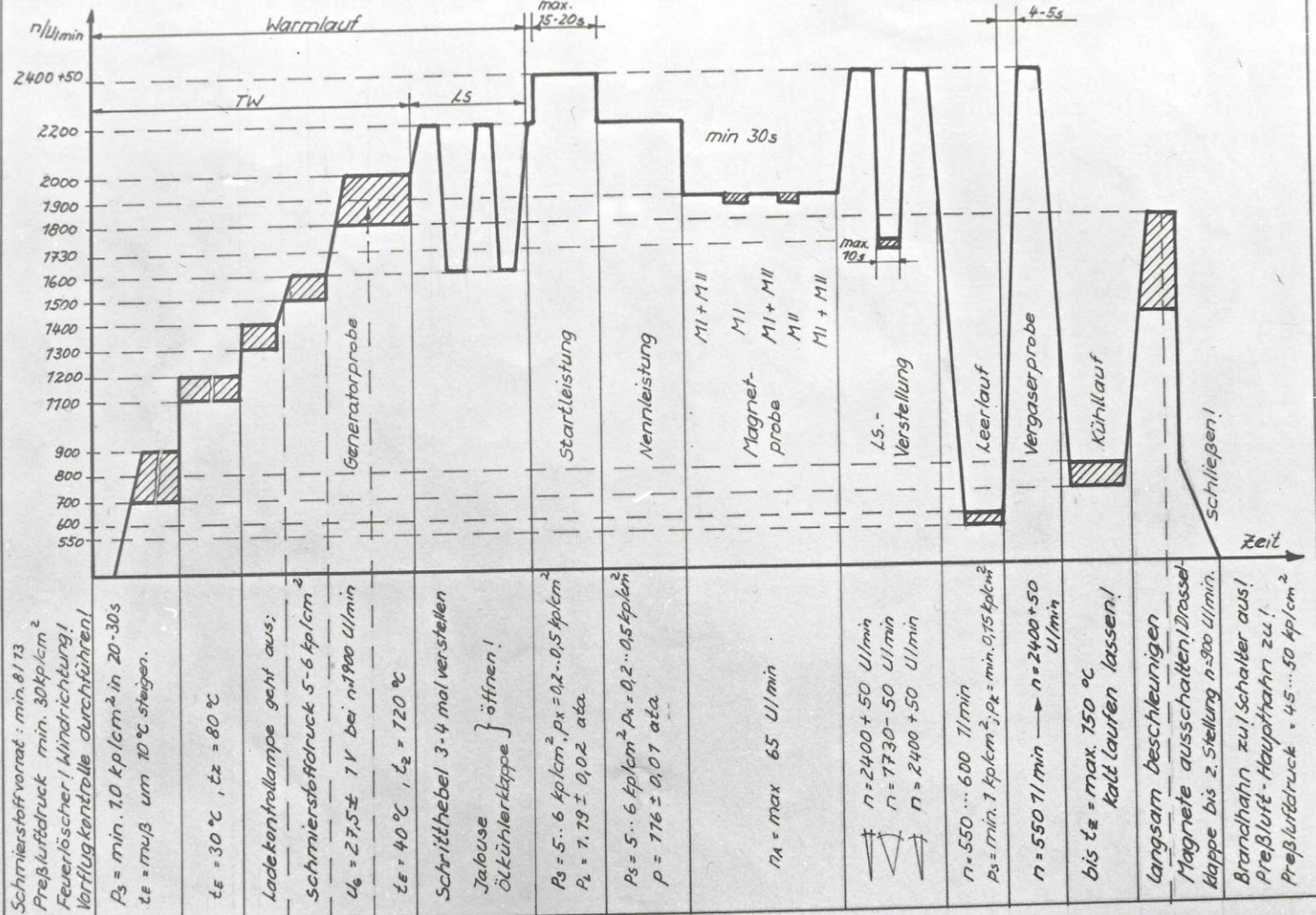
Abbremsdiagramm für M462 RF
